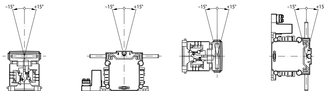
Horizontal assembly «Table mounting»
